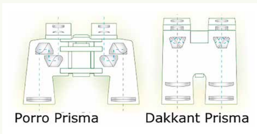
Links een verrekijker met Porroprisma's, rechts een met dakkantprisma's. Bij een verrekijker met Porroprisma's heeft de tubus een opvallende knik en is de optische as verschoven. Een kijker met dakkantprisma's kan je herkennen aan de rechte tubus waarbij de optische as schijnbaar recht door loopt.
