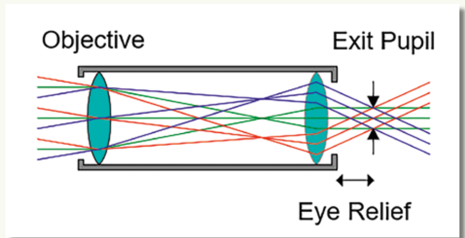
De grootte van de uittredeupil (exit pupil) heb je nodig om de lichtsterkte van een kijker te berekenen. En wat weinig mensen weten: als je een verrekijker gebruikt moet je ook rekening houden met de ideale oogafstand (eye relief)!
